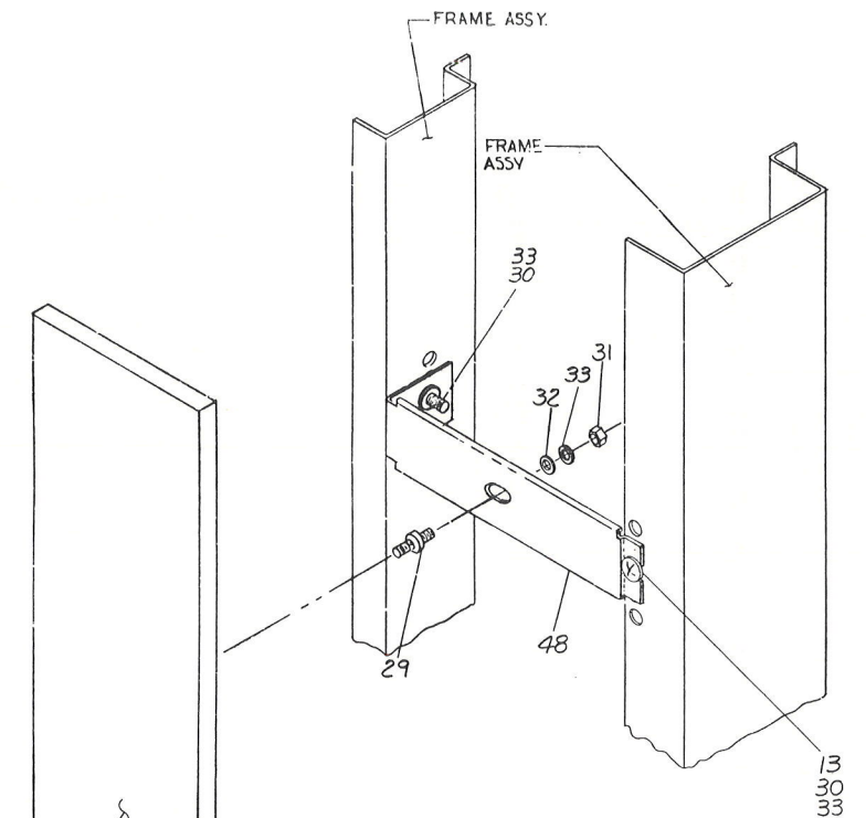
DETAIL C SCALE: NONE
